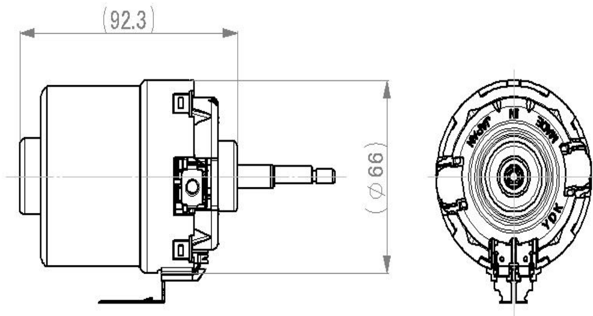
Dimension【mm】
